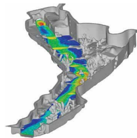
3D model nového kanálu u původního koryta. Dole model s vyznačením toku.
